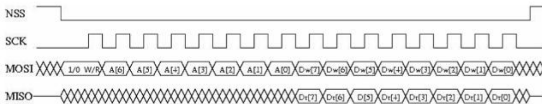
SPI 单地址时序图
