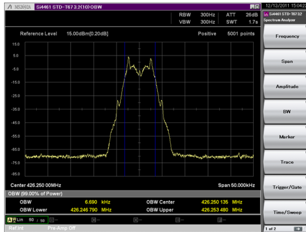
模块发送调制数据图谱
