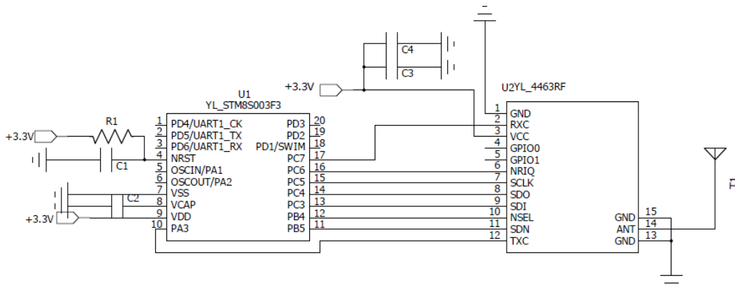
此图基于 STM8S 单片机设计
