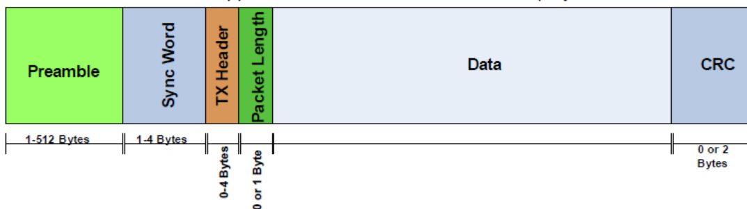
完整包结构图
