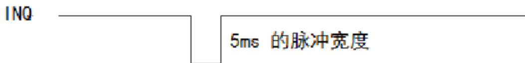
INQ 中断时序
