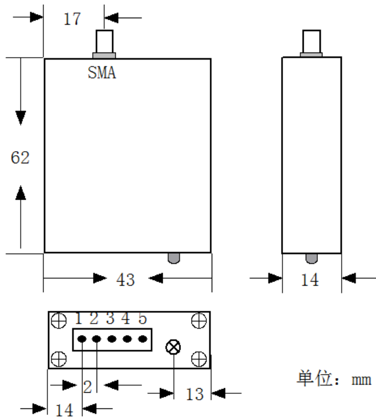
YL-500IW管脚排列图
